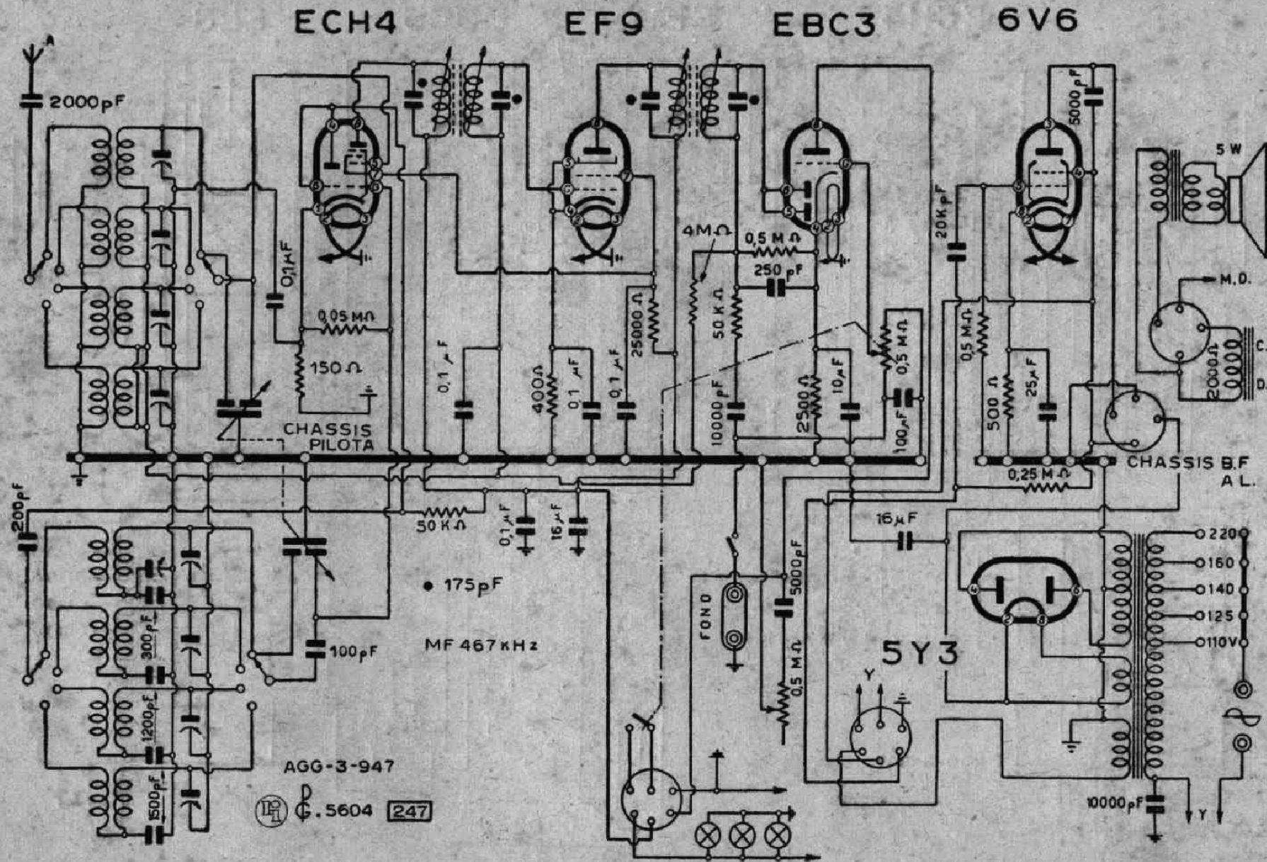
La schema elettrico del mod. 543
